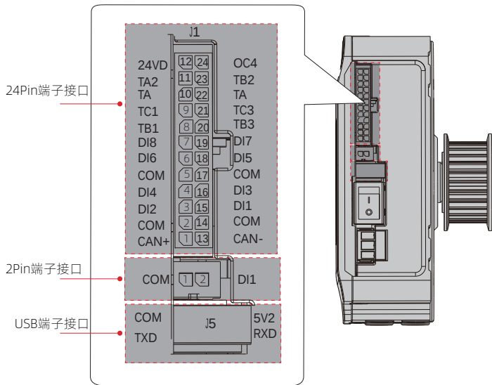
图 3-4 信号端子分布示意图
