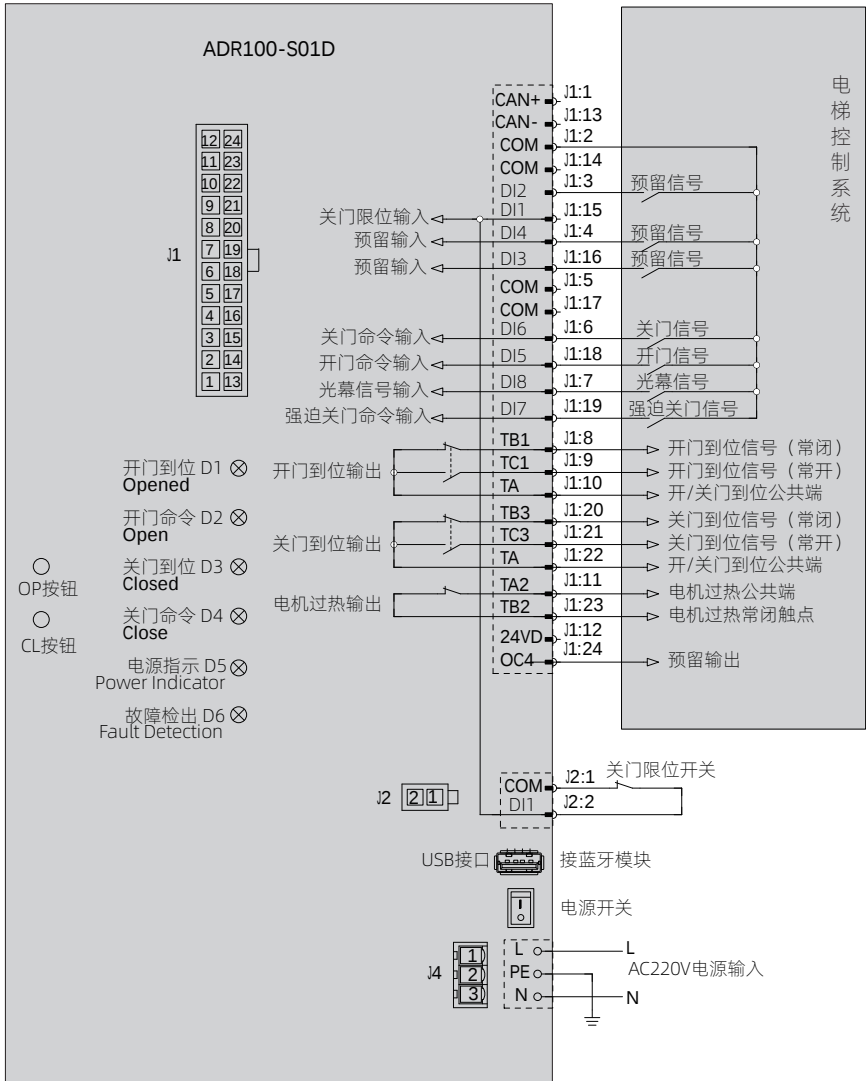
图 3-1 电气接线示意图
