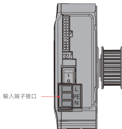
图 3-3 功率端子分布示意图
