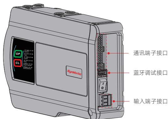
图 3-2 控制器对外接口示意图
