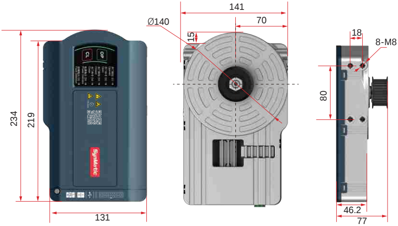
图 2-4 安装尺寸示意图（单位：mm）
