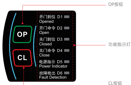
图 4-1 面板按键示意图
