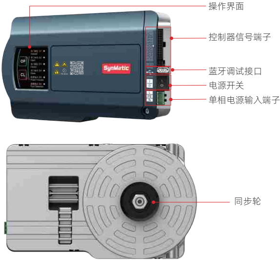
图 1-1 部件说明示意图
