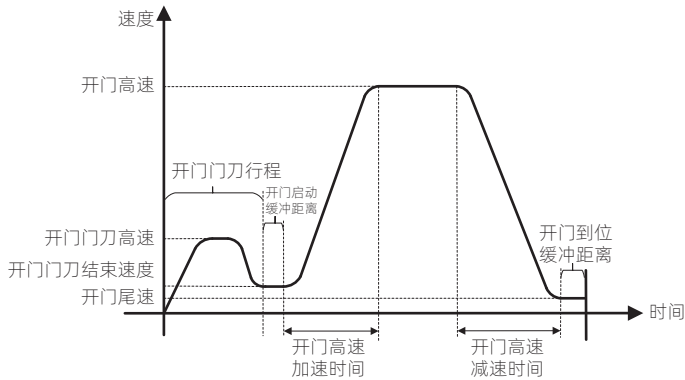
图 5-1 开门曲线
