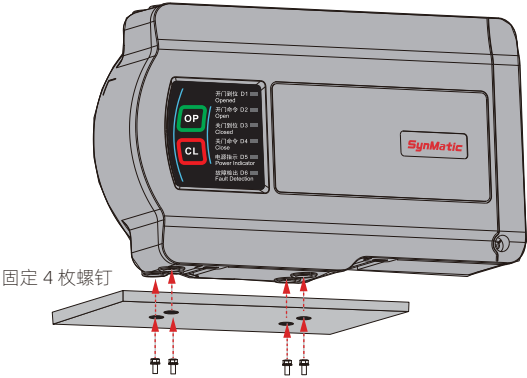
图 2-3 安装方式示意图 2
